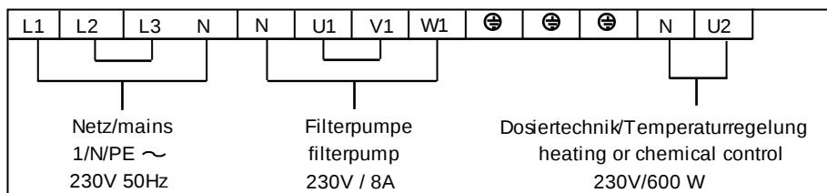
Anschluss einer 230V Wechselstrompumpe
