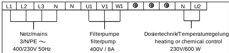
Anschluss einer 400V Drehstrompumpe
